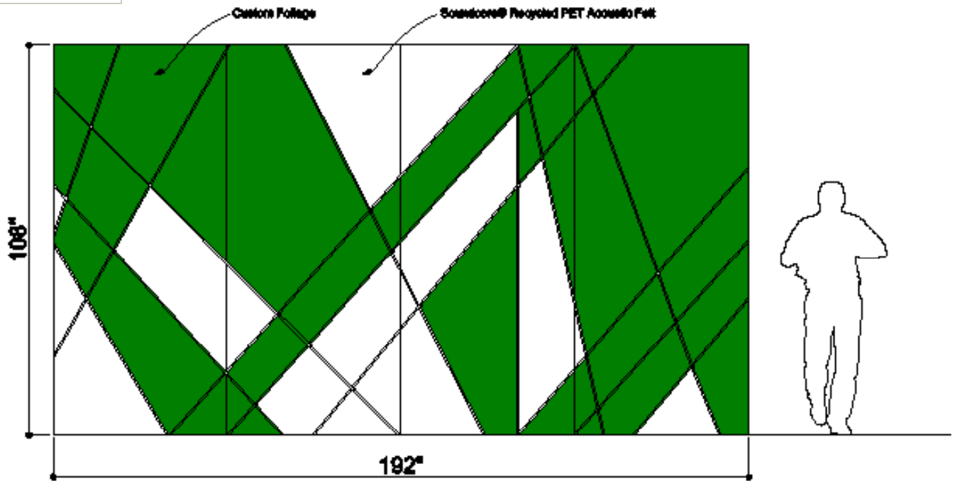
① ELEVATION 1
